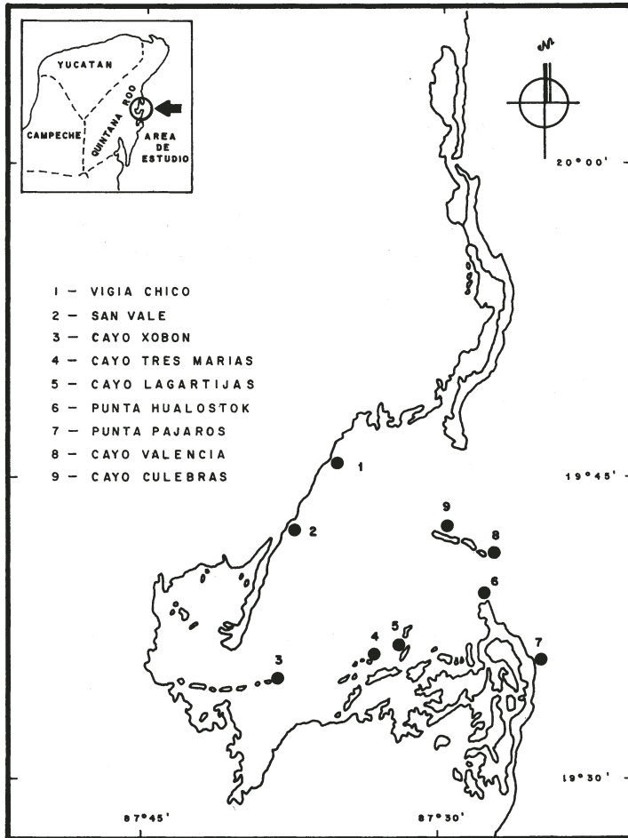
Fig. 2. Localización del área de estudio y sitios de muestreo en la Bahía de la Ascensión, Quintana Roo.
